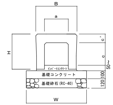
横断用側溝工
