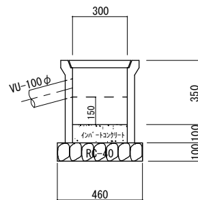
宅地柵 S=1/20
