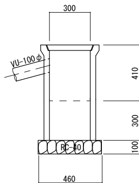
浸透柵詳細図 S=1/20
