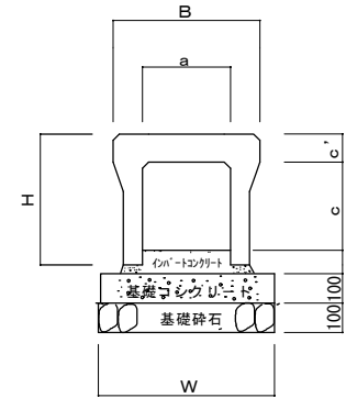
標準用側溝工
