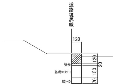
地先境界ブロック工 S=1/20
